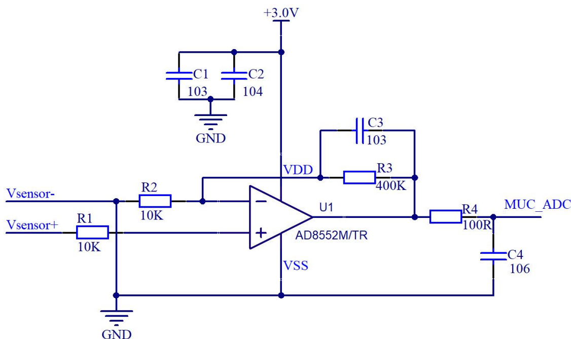
图 3. AO-08 推荐应用电路图
