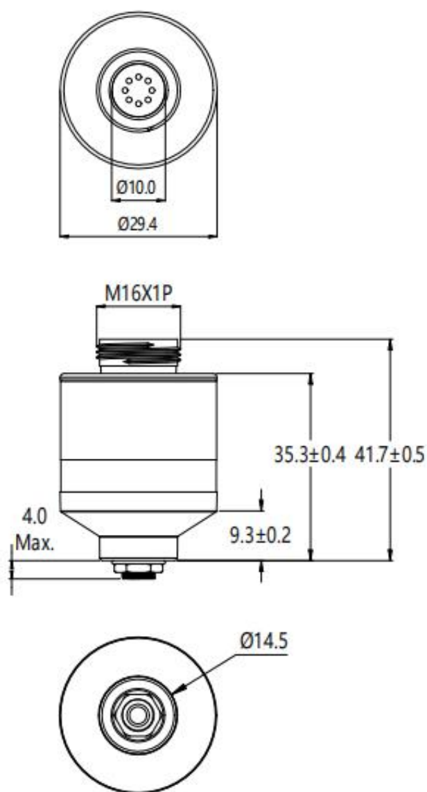
图2. AO-08 外形尺寸图（单位：mm，其他未标注公差： \pm 0.2 \text{ mm} ）
